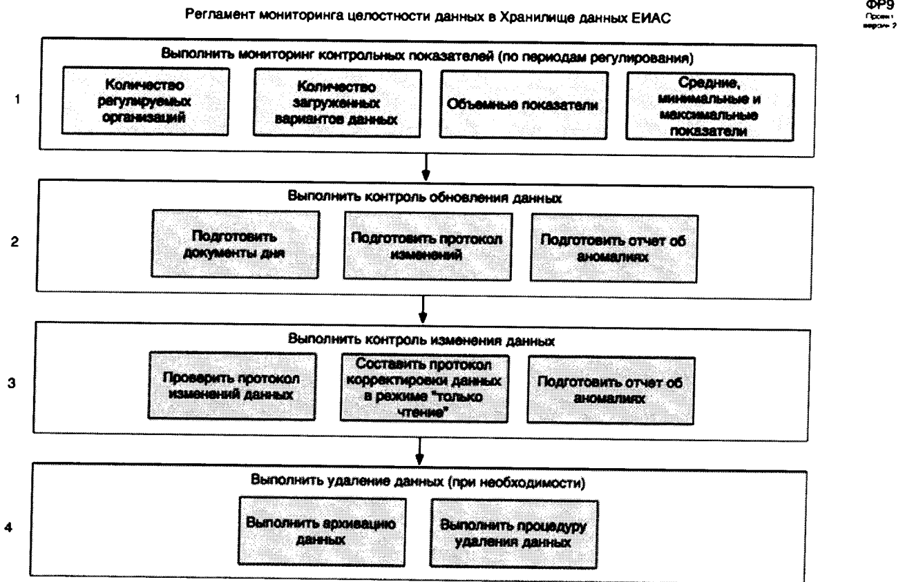
Рис.9 Блок-схема регламента мониторинга целостности данных в Хранилище данных ФГИС ЕИАС ФСТ РФ
