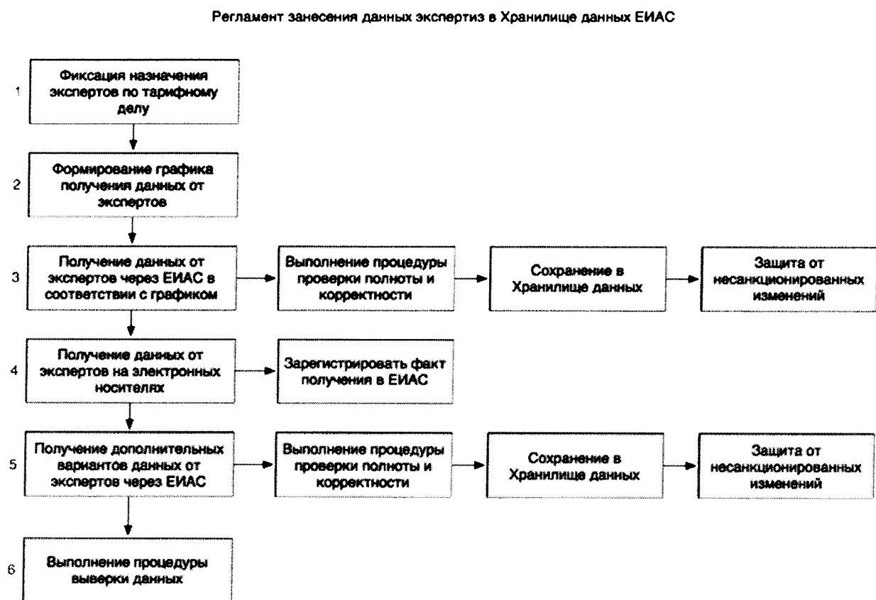
Рис.6 Блок-схема регламента занесения данных экспертиз в Хранилище данных ФГИС ЕИАС ФСТ РФ
