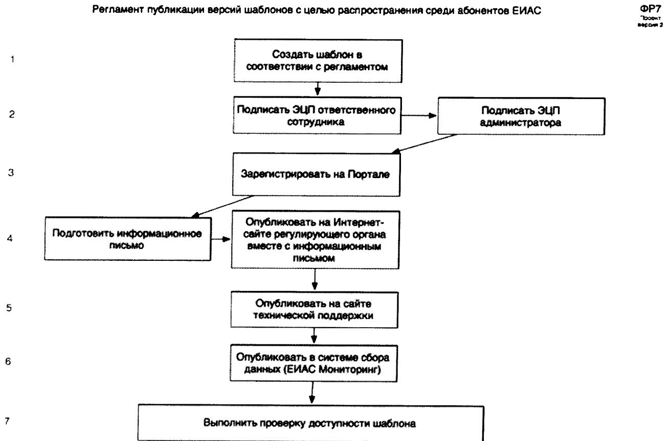
Рис.7 Блок-схема регламента публикации версий шаблонов с целью распространения среди абонентов ФГИС ЕИАС ФСТ РФ
