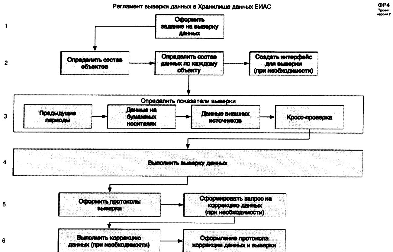
Рис.4 Блок-схема регламента выверки данных в Хранилище данных ФГИС ЕИАС ФСТ РФ
