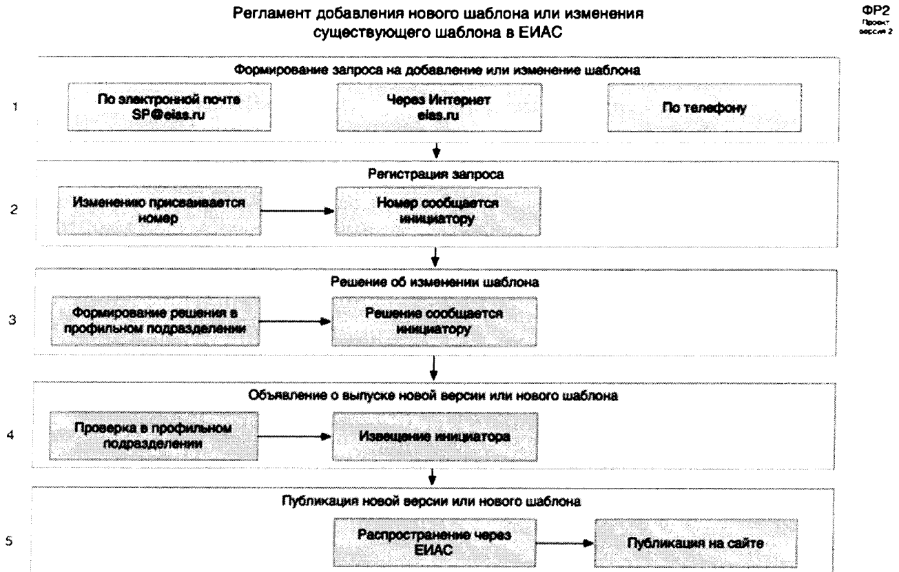
Рис.2 Блок-схема регламента добавления нового шаблона или изменения существующего шаблона в ФГИС ЕИАС ФСТ РФ
