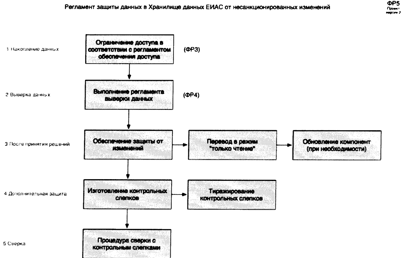
Рис.5 Блок-схема регламента защиты данных в Хранилище данных ФГИС ЕИАС ФСТ РФ от несанкционированных изменений
